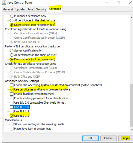
Şekil 4: Java TLS ayarları seçimi
